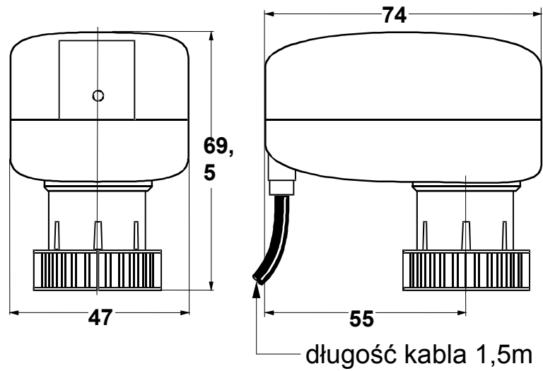
Siłownik VA-7450
