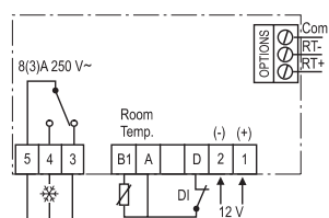
MR42PM12R-1C Wiring
